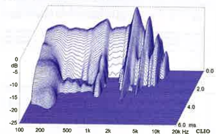
Zerfallspektrum (Wasserfall)
